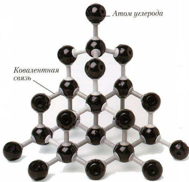
СТРУКТУРА АЛМАЗА
