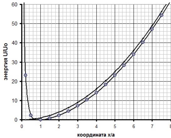
Приближение больших колебаний
