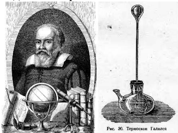
Рис. 30. Термоскоп Галилея
