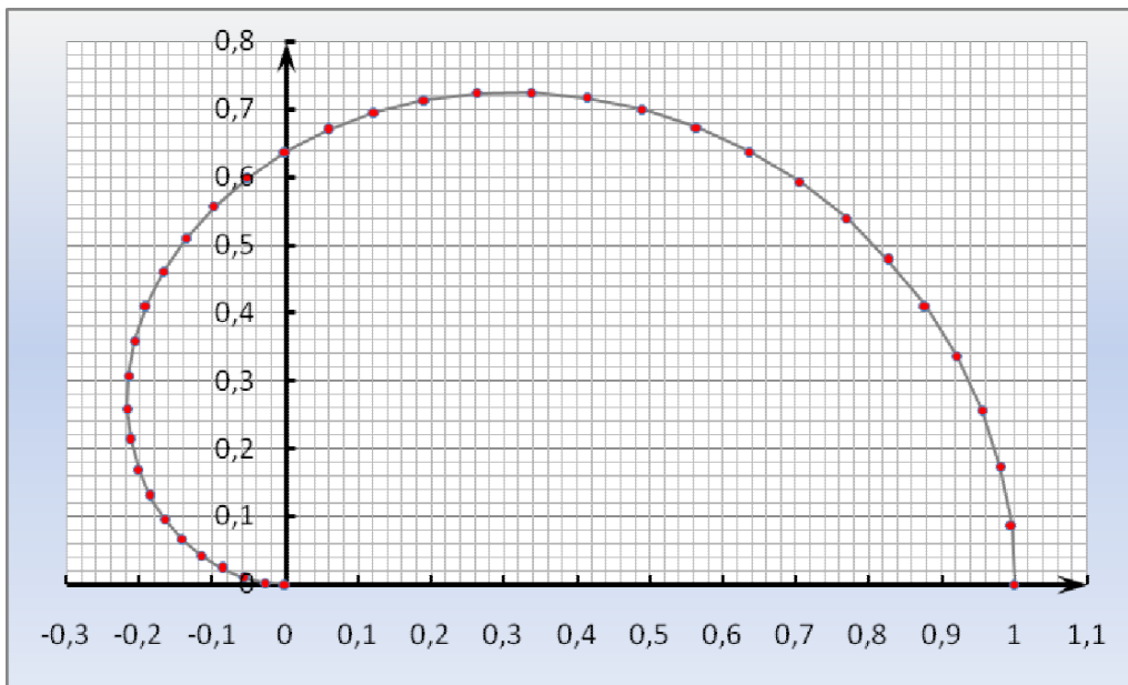
Рис. 6. Траектория центра масс при горении
