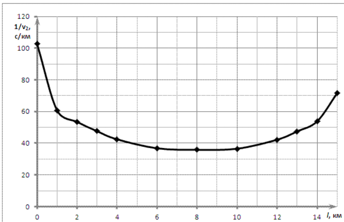
Рисунок 4 - График зависимости обратной скорости от пройденного пути
