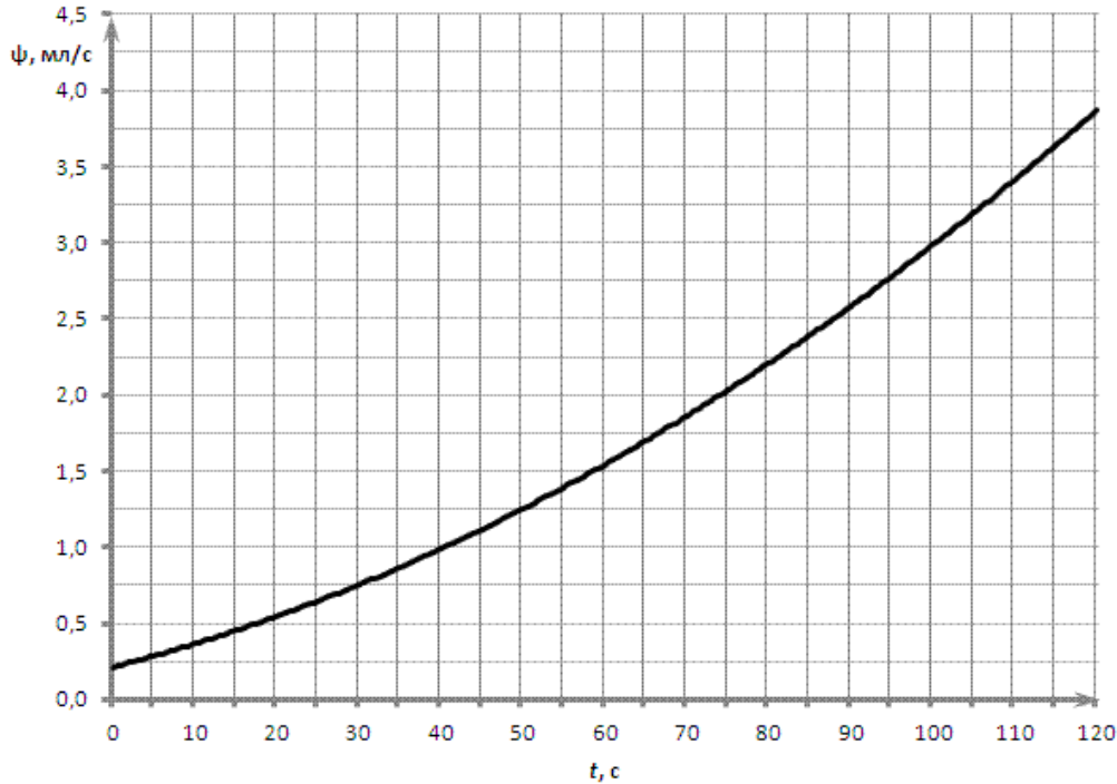
Рисунок 3 - График зависимости временного расхода от времени
