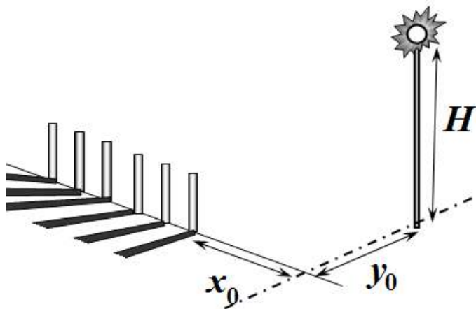
Рис. 1. Геометрия эксперимента.
